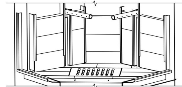
Схема установки трубок дожига «Сибирь-15»
