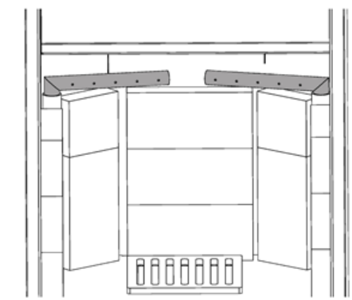
Схема установки трубок дожига «Сибирь-12»
